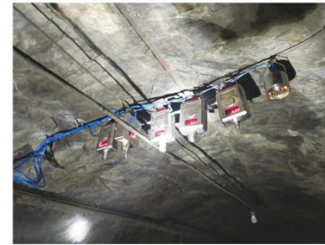
井下总回风巷在线监测系统
