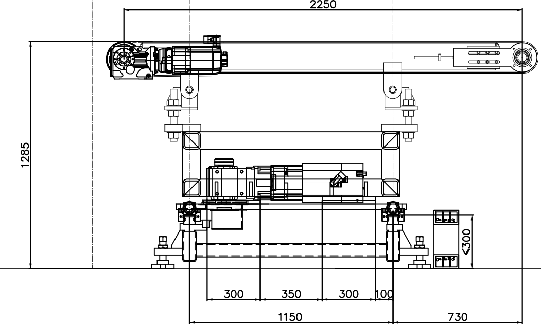
侧移皮带机侧视图
