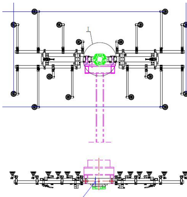
对中端拾器、端拾器更换支架示意图
