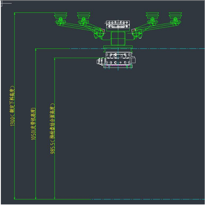
穿梭车、皮带机、下料相对位置示意
