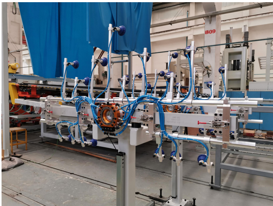
对中端拾器、端拾器更换支架参考图
