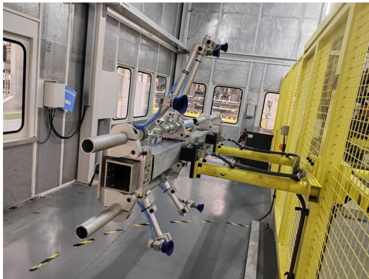
端拾器在旋转门上
