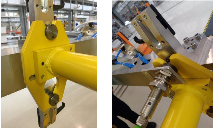
端拾器固定支架及在位检测（仅供参考）
