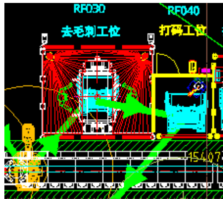
图 1 打码工位布局图
