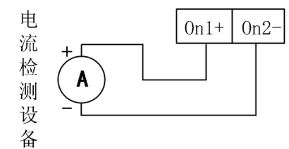
变送输出接线
