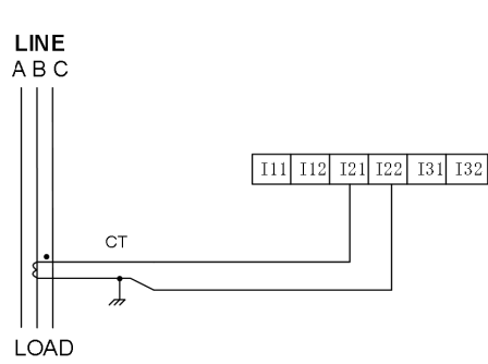
单相电流1CT
