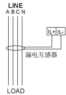
三相四线漏电互感器接线
