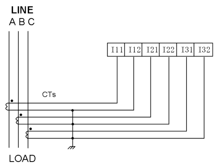
三相3CT(适用于3LN, 3LL)
