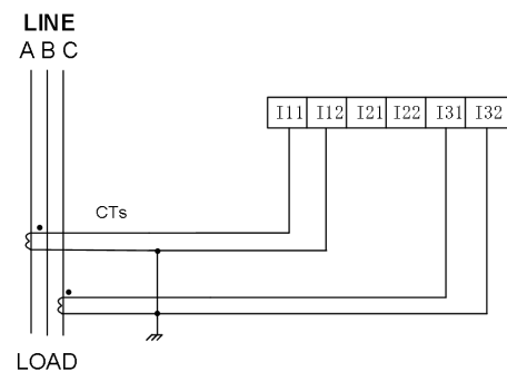
三相2CT直接连接(仅适用于2LL) 高精度仪表不适用
