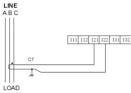
单相电流1CT
