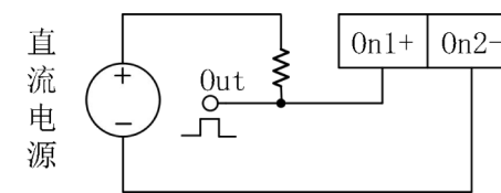
电能脉冲输出接线
