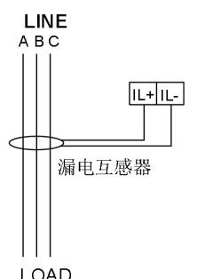
三相三线漏电互感器接线
