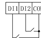
开关量输入接线图
