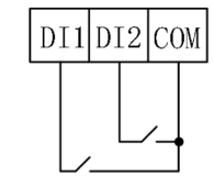
开关量输入接线图
