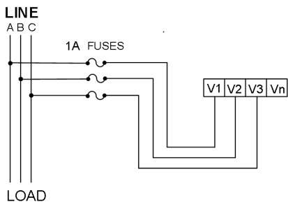
三相三线直接连接(3LL), 低压 (不适用于高精度仪表)
