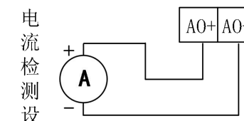
变送输出接线
