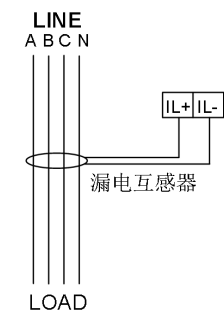
三相四线漏电互感器接线
