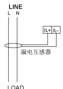
单相漏电互感器接线
