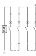
4P 外形 4 极串 3
