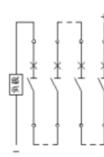
4P 外形 4 极串 3
