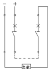
2P 外形 2 极串 2
