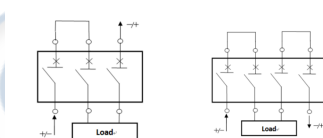
三极串 接线图
