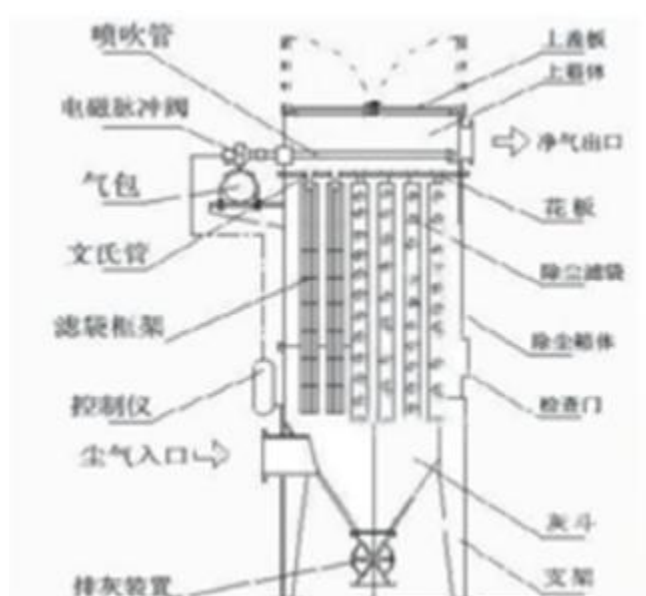
图 10.2-5 布袋除尘器工作原理
