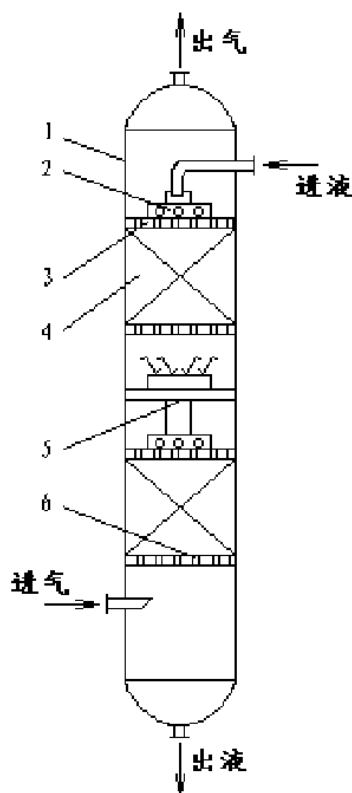
1-塔壳体；2-液体分布器；3-填料压板；4-填料；5-液体再分布装置；6-填料支撑板
