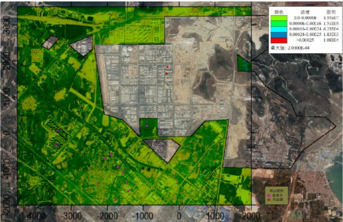
图 6.1-8 本项目 NO x 年均值浓度贡献值分布图
