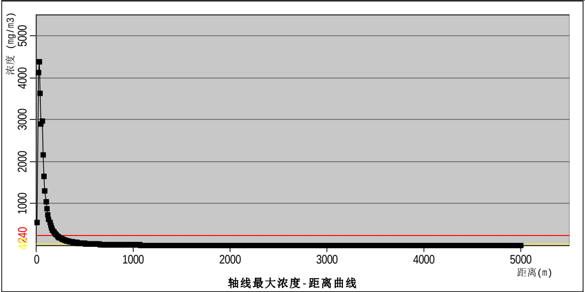
图 7.9-6 MDI 扩散轴线最大浓度曲线图 最常见气象条件下 MDI 储罐泄漏 MDI 扩散预测浓度达到不同毒性终点浓度的最大影响范围见图 7.9-7。
