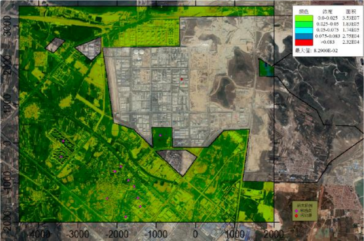
图 6.1-28 非正常工况下 NO x 小时浓度贡献值分布图
