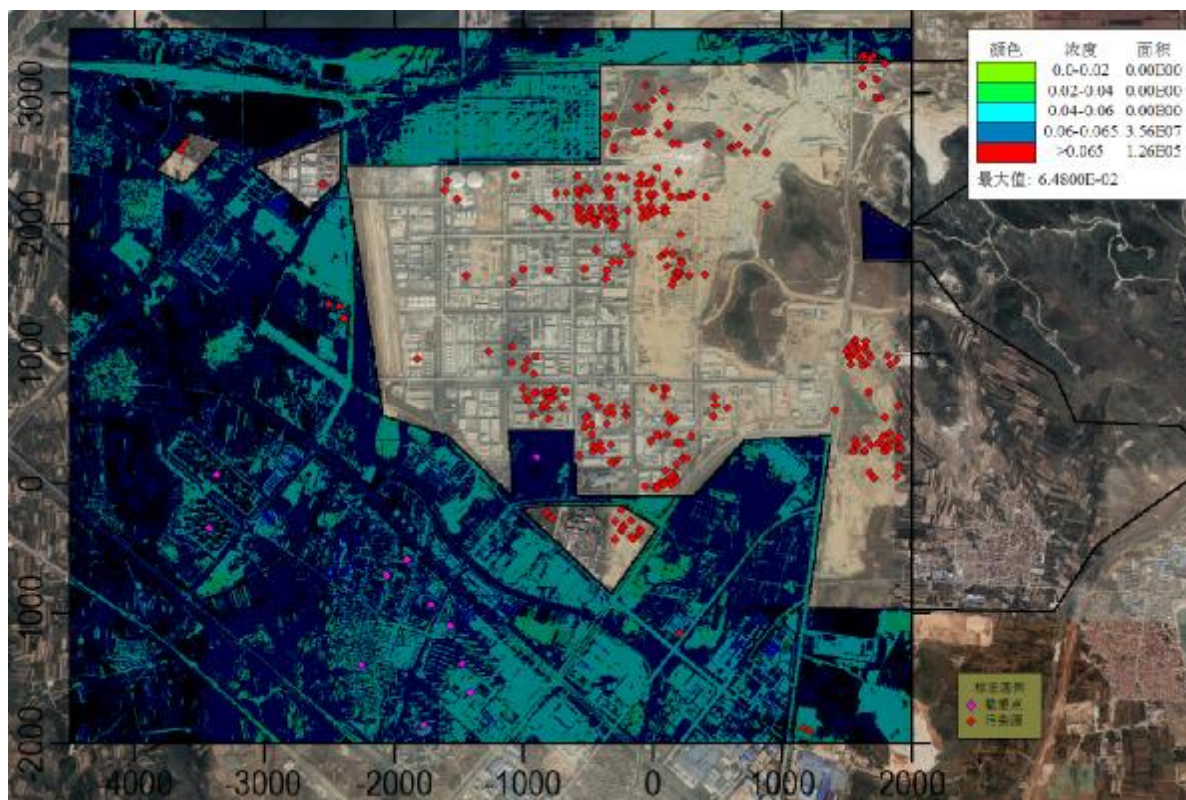
图 6.1-26 叠加后 PM 2.5 95%保证率日均环境质量浓度预测分布图
