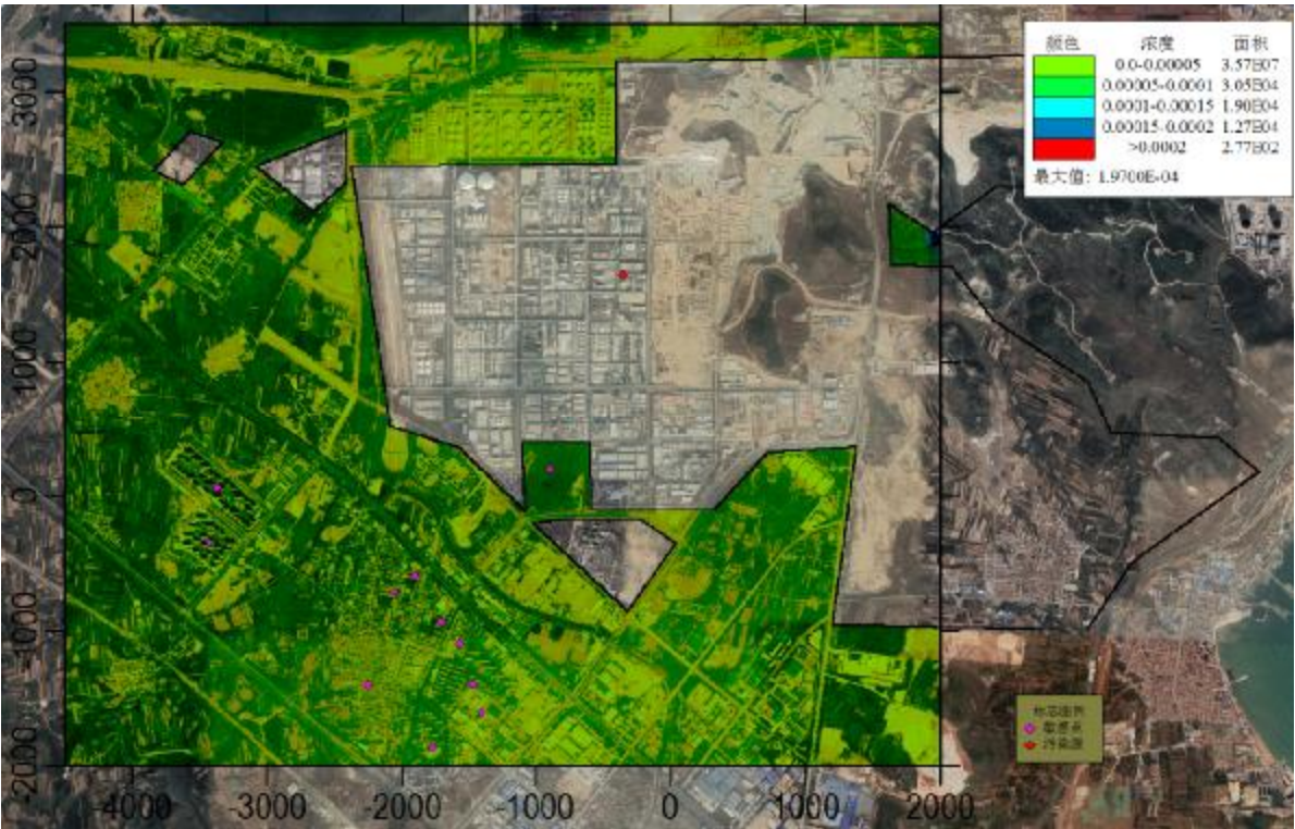
图 6.1-18 本项目合并排放后 PM 10 年均值浓度贡献值分布图
