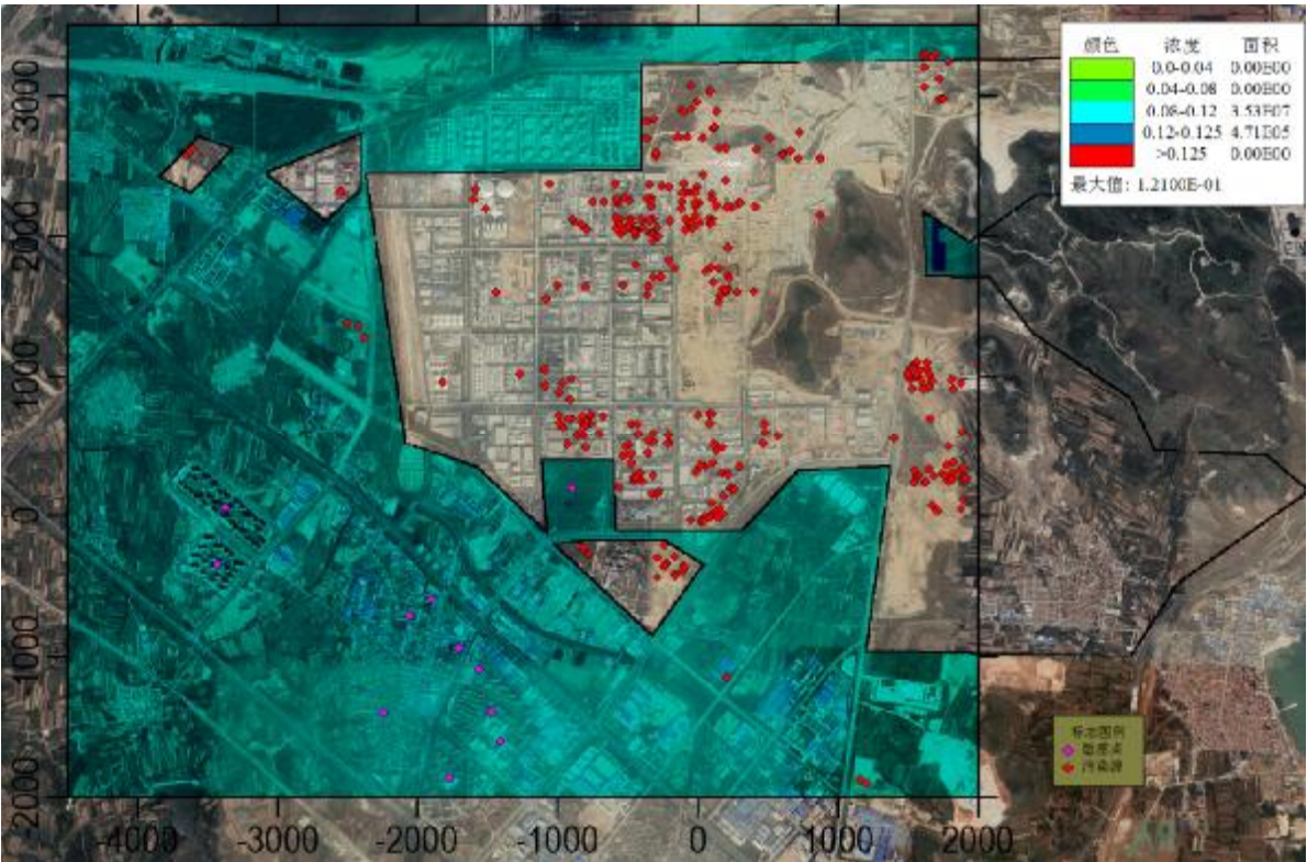
图 6.1-24 叠加后 PM 10 95% 保证率日均环境质量浓度预测分布图
