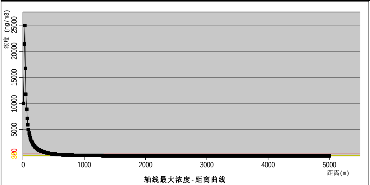
图 7.9-1 丁酮储罐泄漏燃烧次生 CO 扩散轴线最大浓度曲线图 最不利气象条件下丁酮储罐泄漏燃烧次生 CO 扩散预测浓度达到不同毒性终点浓
