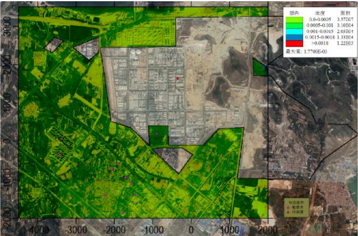
图 6.1-17 本项目合并排放后 PM 10 日均值浓度贡献值分布图
