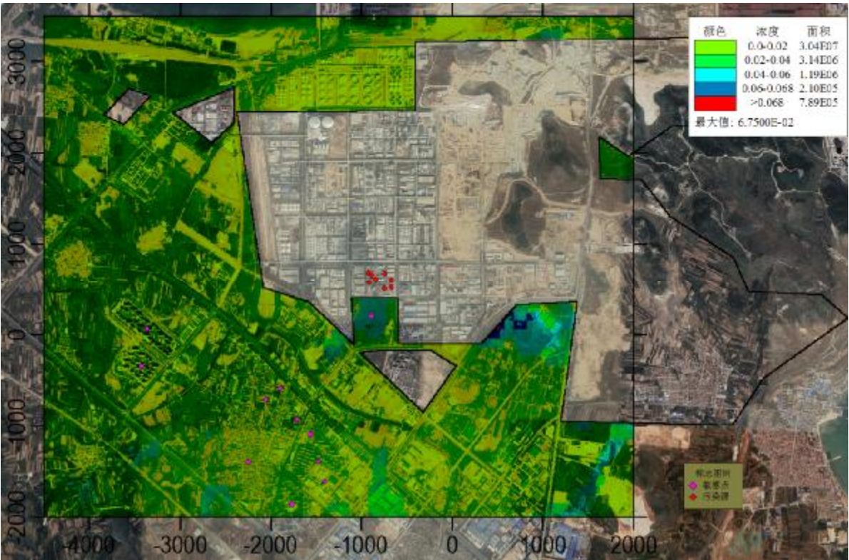
图 6.1-9 本项目 VOCs 小时值浓度贡献值分布图
