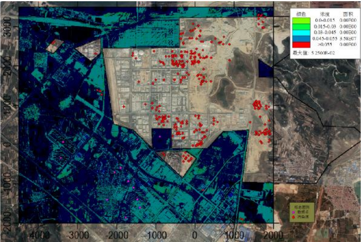
图 6.1-25 叠加后 PM 10 年均环境质量浓度预测分布图
