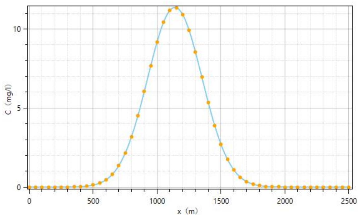
图 6.3-10 瞬时泄漏泄漏点处 COD Cr 浓度变化图（3650d）
