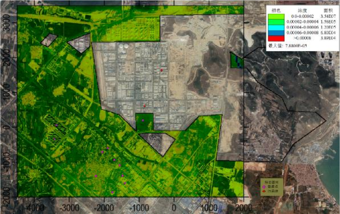
图 6.1-12 本项目 PM 2.5 日均值浓度贡献值分布图
