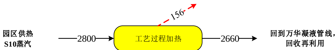
图 3.4-1 拟建项目蒸汽平衡图 (t/a)
