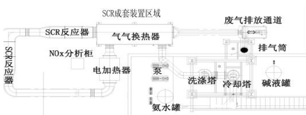
图 10.2-4 SCR 废气处理系统工艺流程图
