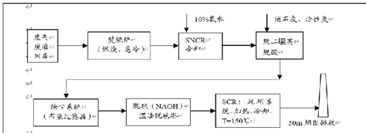
图 10.2-7 依托的 TDI 能量回收焚烧炉工艺流程框图
