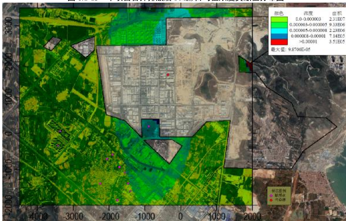
图 6.1-20 本项目合并排放后 PM 2.5 年均值浓度贡献值分布图
