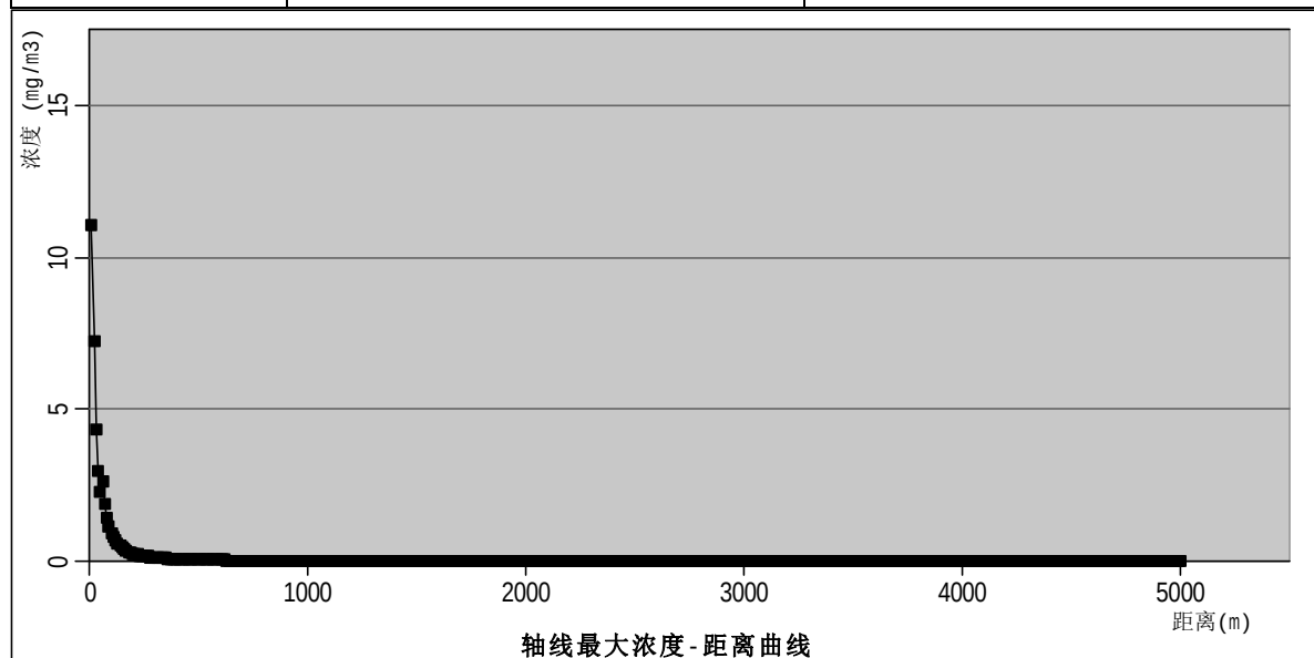
图 7.9-3 丁酮储罐泄漏燃烧次生 CO 扩散轴线最大浓度曲线图
