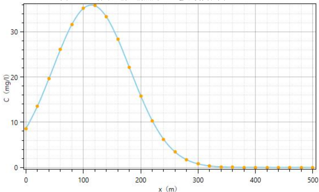
图 6.3-9 瞬时泄漏泄漏点处 \text{COD}_{\text{Cr}} 浓度变化图 (365d)
