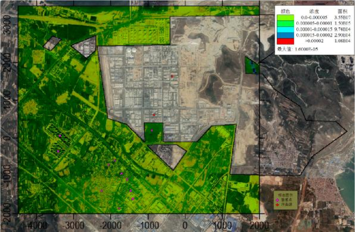
图 6.1-11 本项目 PM 10 年均值浓度贡献值分布图
