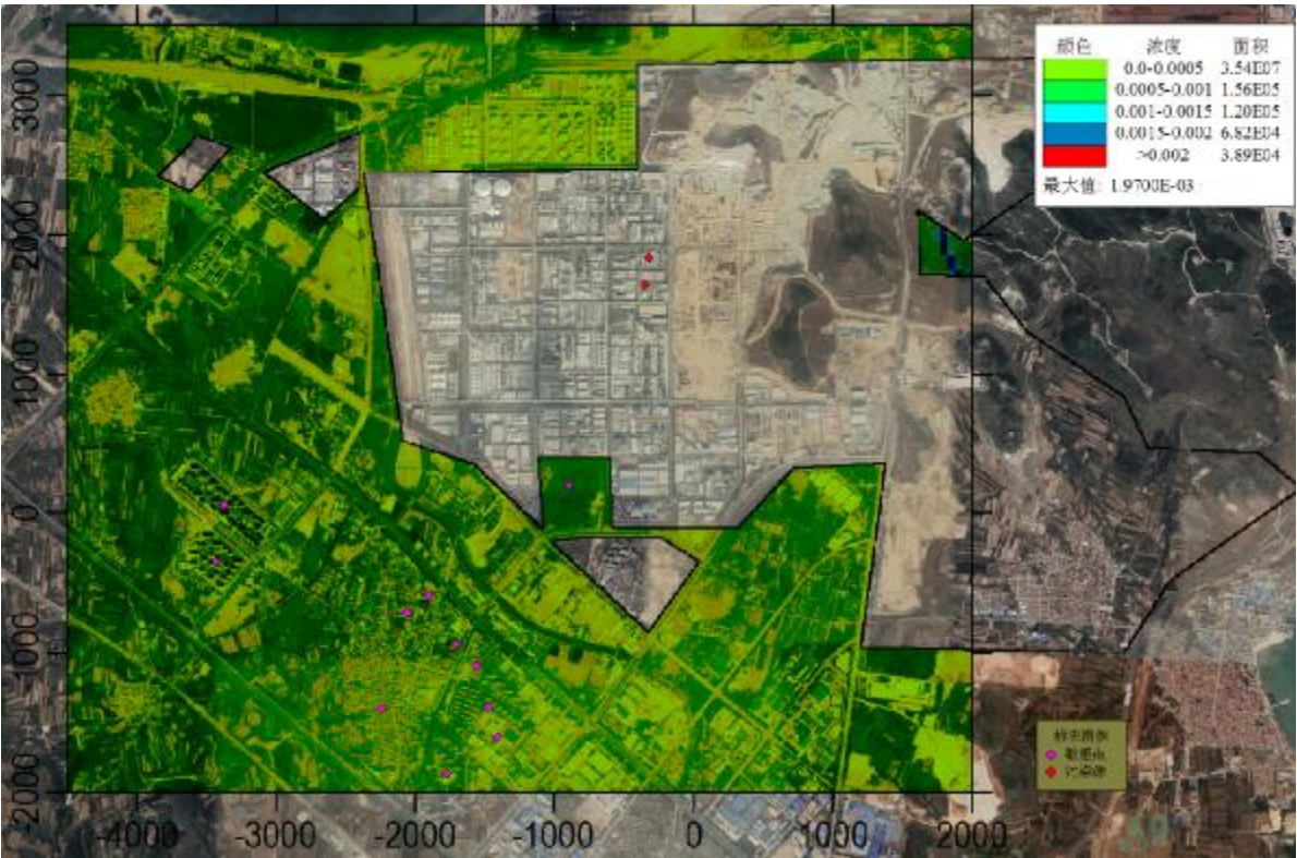
图 6.1-7 本项目 NO x 日均值浓度贡献值分布图
