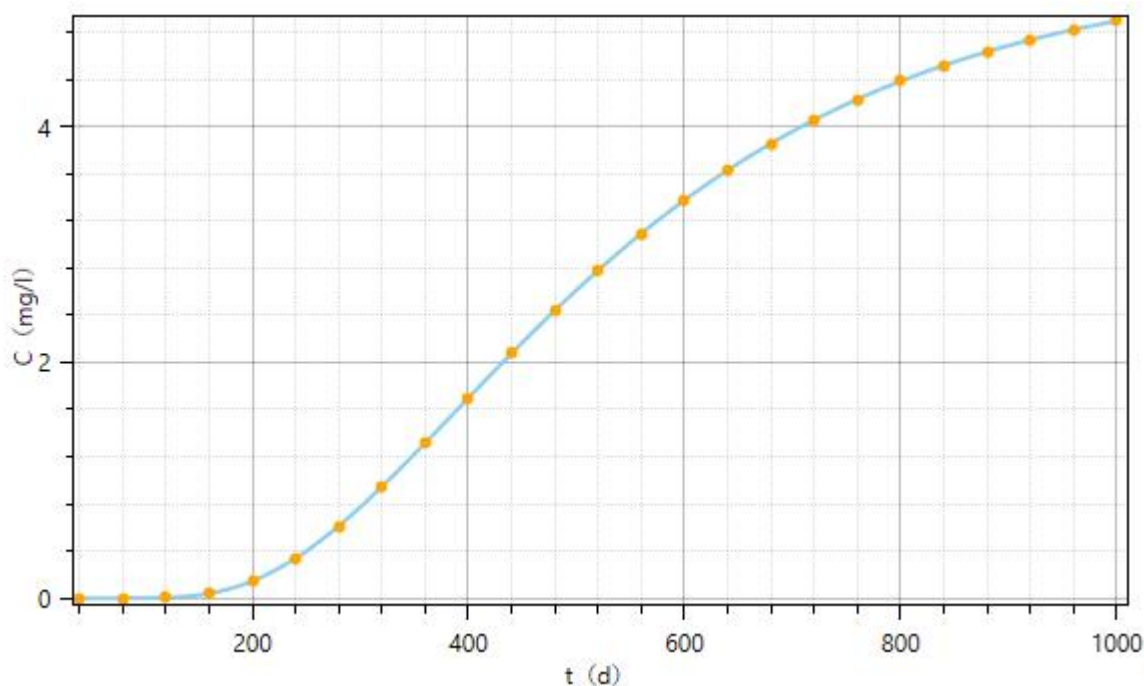
图 6.3-11 连续泄漏泄漏点下游 COD Cr 的浓度变化情况图
