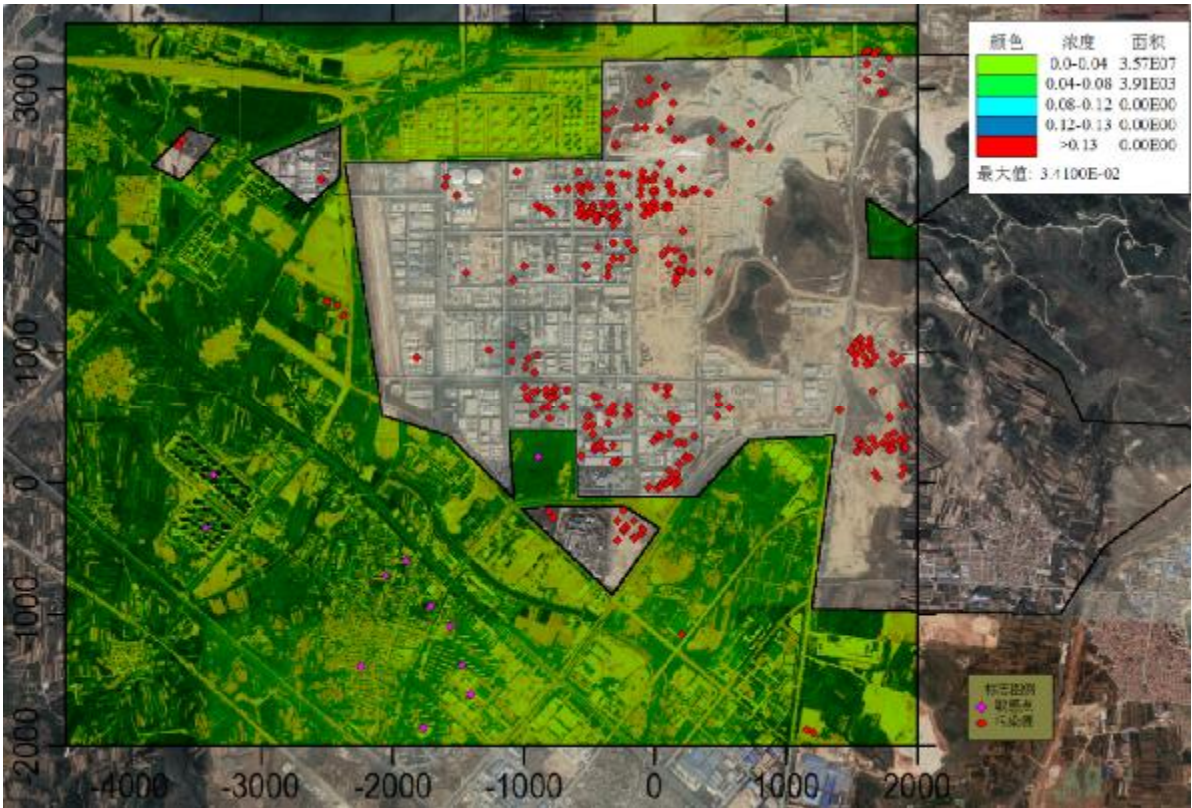
图 6.1-22 叠加后 NO x 年均环境质量浓度预测分布图
