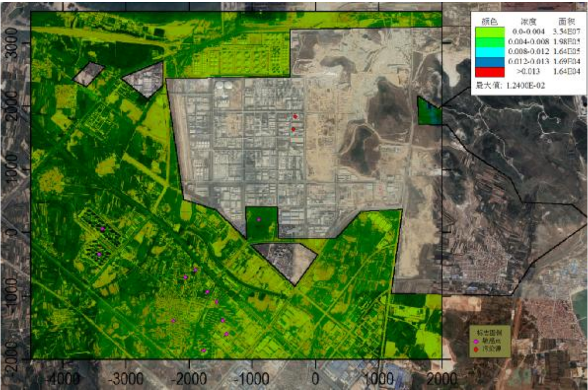
图 6.1-6 本项目 NO x 小时值浓度贡献值分布图
