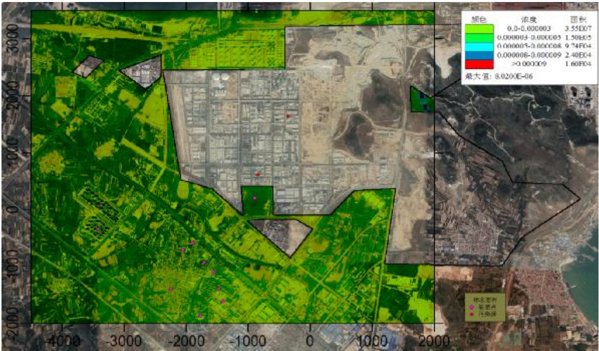
图 6.1-13 本项目 PM 2.5 年均值浓度贡献值分布图
