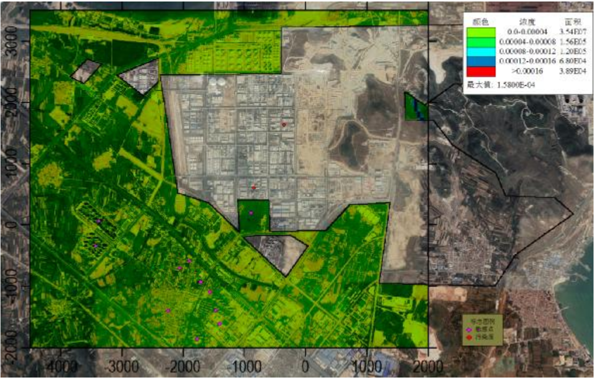
图 6.1-10 本项目 PM 10 日均值浓度贡献值分布图
