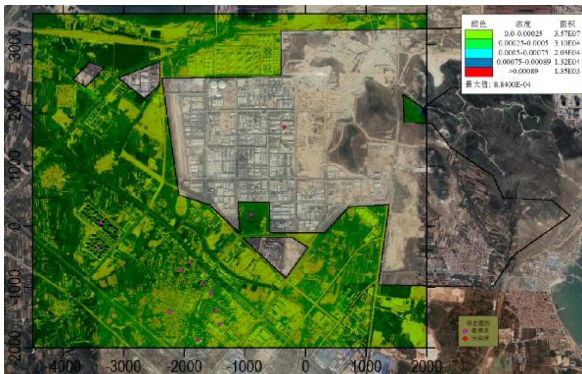
图 6.1-19 本项目合并排放后 PM 2.5 日均值浓度贡献值分布图
