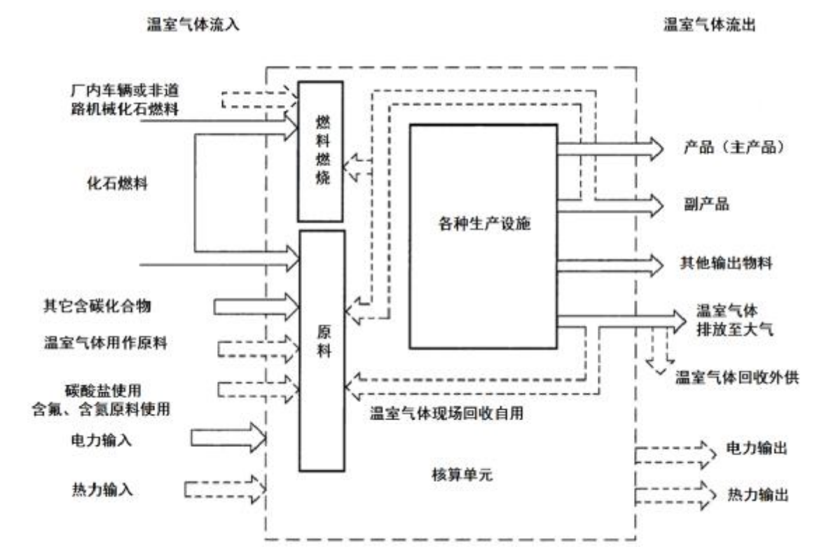
图 8.3-1 化工行业温室气体源流识别示意图
