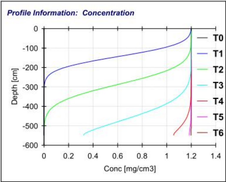
图 6.7-3 不同渗漏时间铜盐影响深度和浓度示意图
