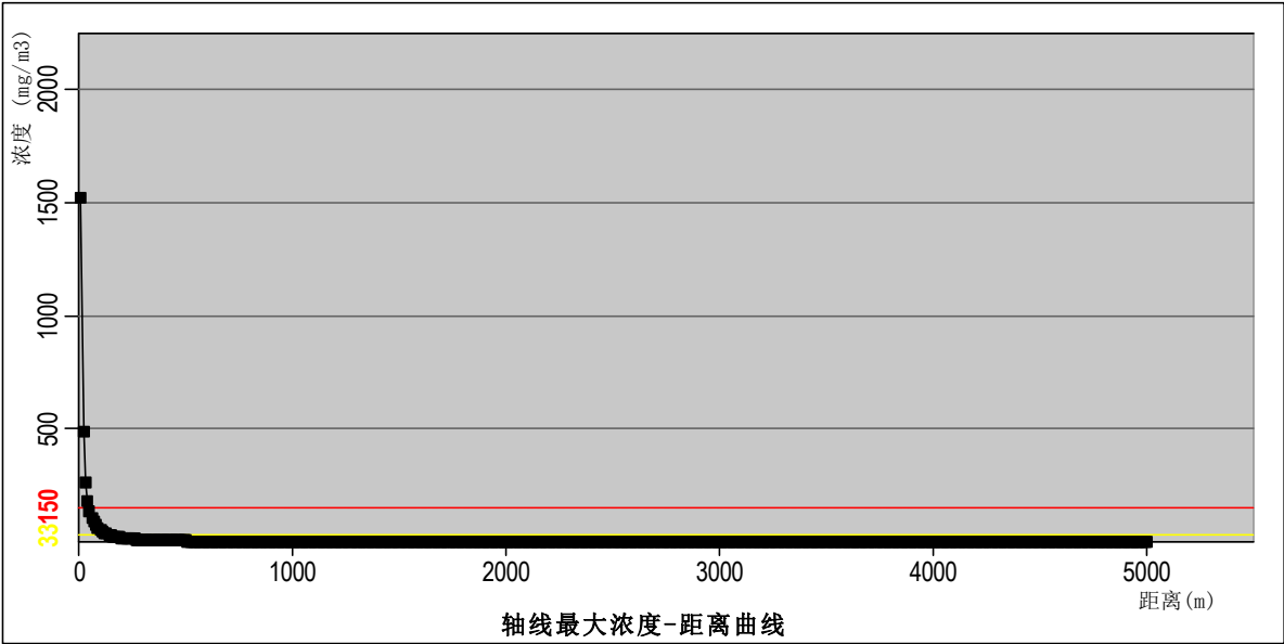
图 7.9-3 盐酸储罐泄漏 HCl 扩散轴线最大浓度曲线图 最不利气象条件下盐酸储罐泄漏 HCl 扩散预测浓度达到不同毒性终点浓度的最大影响范围见图 7.9-4。
