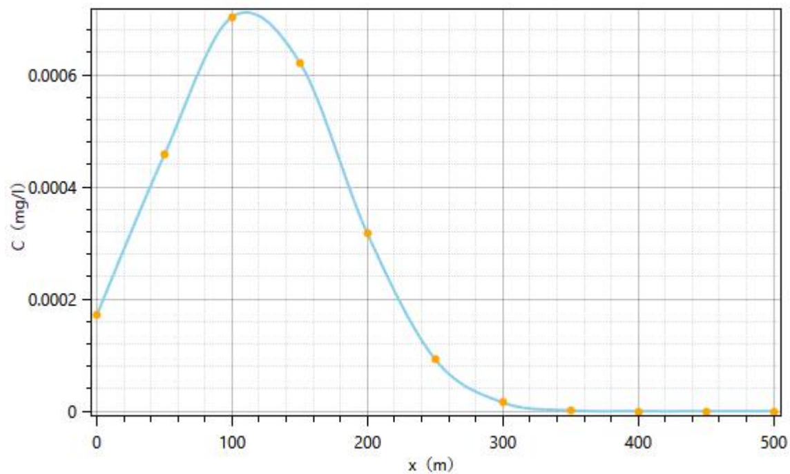
图 6.3-9 瞬时泄漏泄漏点处 COD Cr 浓度变化图（365d）
