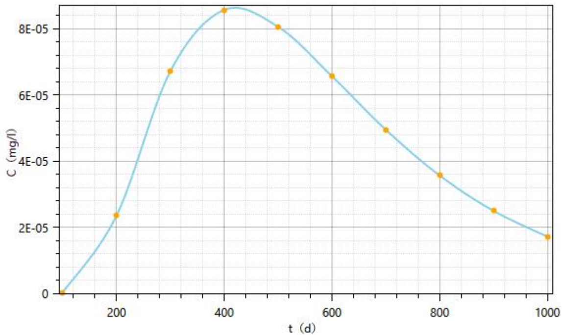
图 6.3-14 连续泄漏泄漏点下游 COD Cr 的浓度变化情况图
