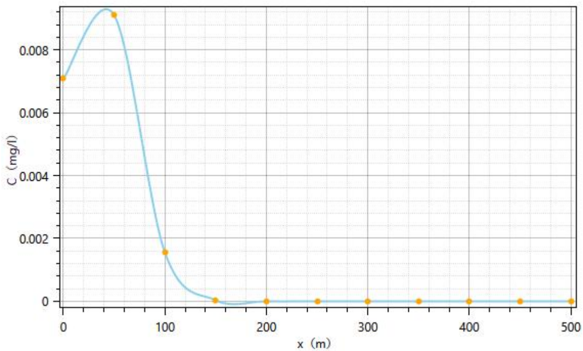
图 6.3-11 瞬时泄漏泄漏点处铜离子浓度变化图（100d）
