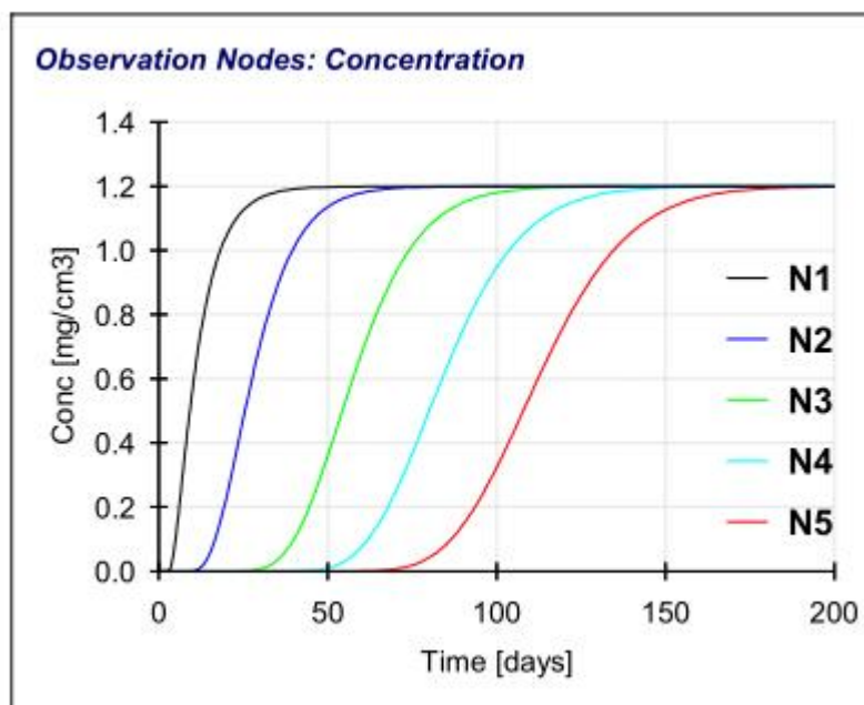
图 6.7-2 包气带各观测点铜盐浓度随时间变化示意图
