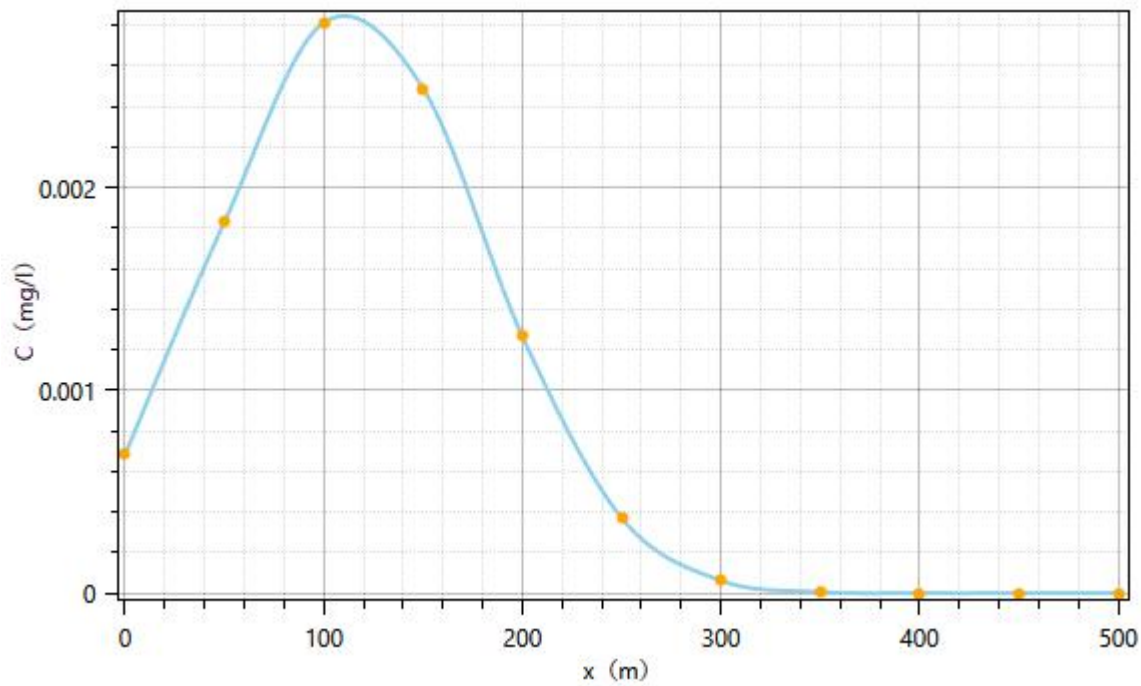
图 6.3-12 瞬时泄漏泄漏点处铜离子浓度变化图（365d）
