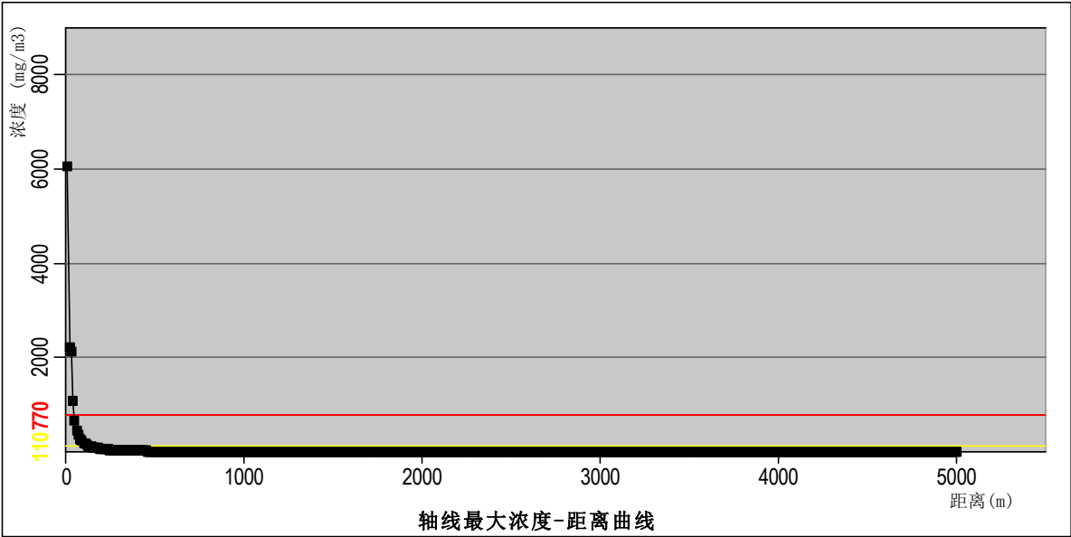
图 7.9-5 氨水储罐泄漏 NH 3 扩散轴线最大浓度曲线图 最不利气象条件下，氨水储罐泄漏 NH 3 扩散预测浓度达到不同毒性终点浓度的最大影响范围见图 7.9-6。
