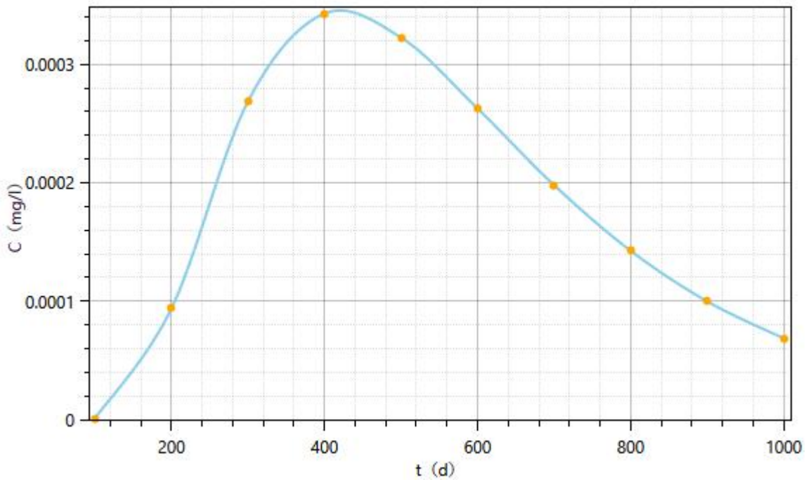
图 6.3-15 连续泄漏泄漏点下游铜离子的浓度变化情况图
