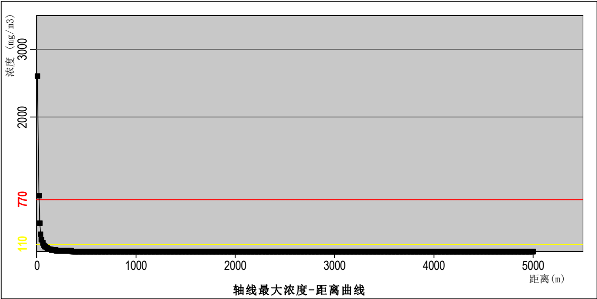
图 7.9-7 氨水储罐泄漏 NH 3 扩散轴线最大浓度曲线图
