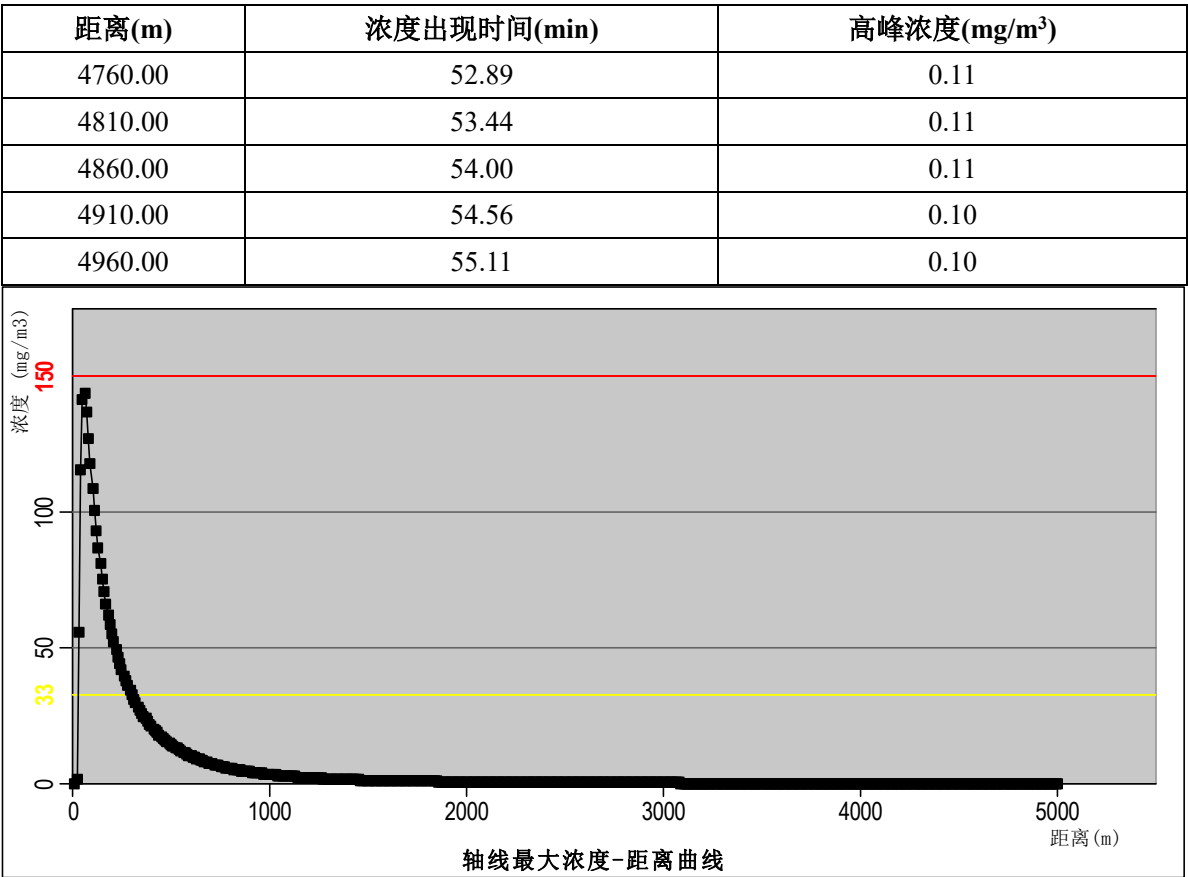
图 7.9-1 盐酸储罐泄漏 HCl 扩散轴线最大浓度曲线图 最不利气象条件下盐酸储罐泄漏 HCl 扩散预测浓度达到不同毒性终点浓度的最大影响范围见图 7.9-2。
