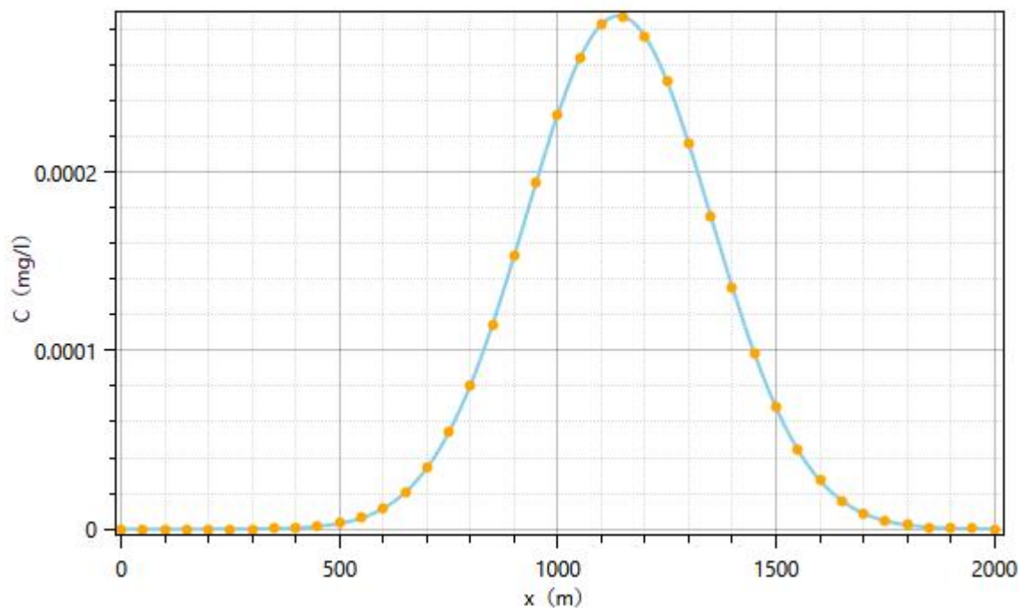
图 6.3-13 瞬时泄漏泄漏点处铜离子浓度变化图（3650d） 表 6.3-7 瞬时渗漏时污染物影响预测结果表
