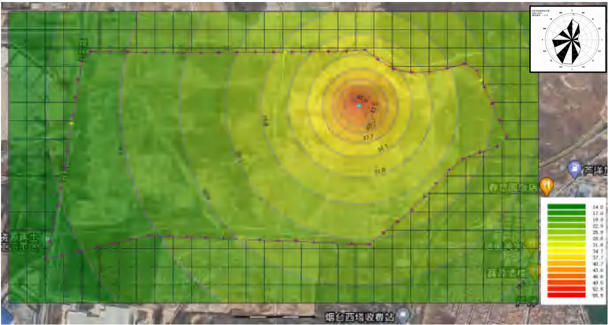
图 6.5-1 本技改项目噪声贡献值预测结果
