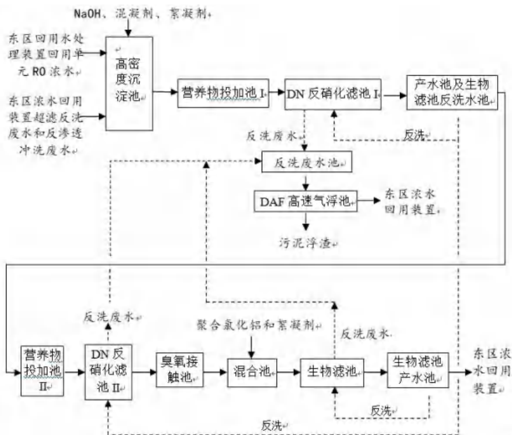
图 7.2-7 浓水处理装置工艺流程示意图 (a)
