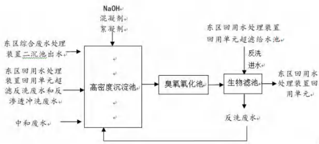
图 7.2-5 回用水处理装置预处理单元工艺流程示意图
