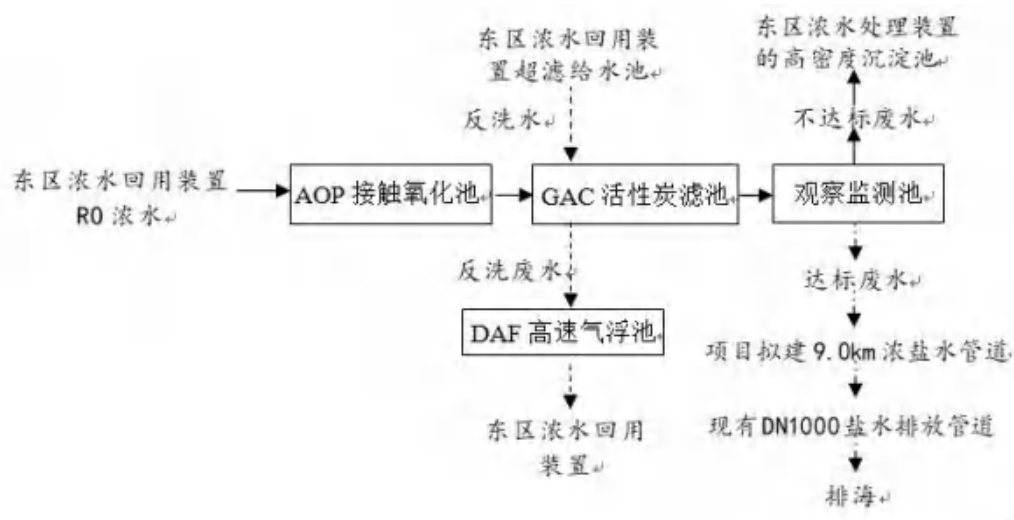
图 7.2-8 浓水处理装置工艺流程示意图 (b)
