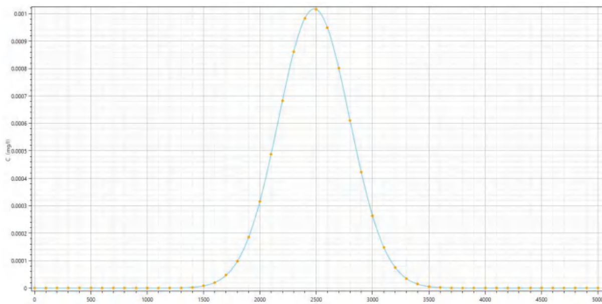
图 6.4-16 20 年后地下水二甲苯浓度和距离关系图
