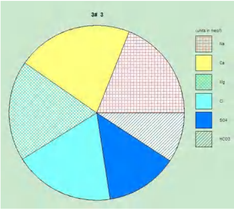
图 6.4-6 地下水水化学常规离子含量对比图
