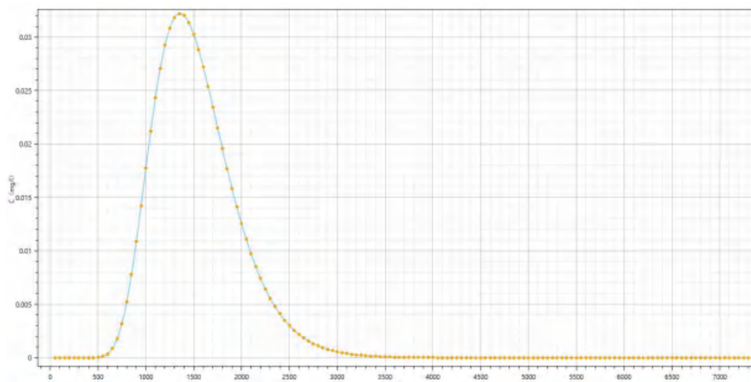
图 7.6-6 厂界浓度随时间变化关系图
