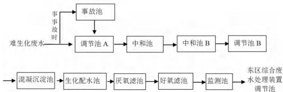
图 7.2-3 难生化废水处理装置工艺流程示意图
