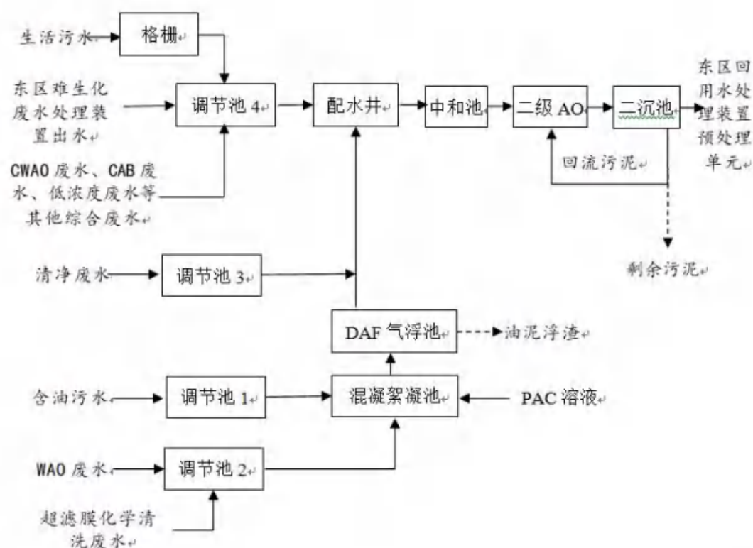
图 7.2-4 综合废水处理装置工艺流程示意图
