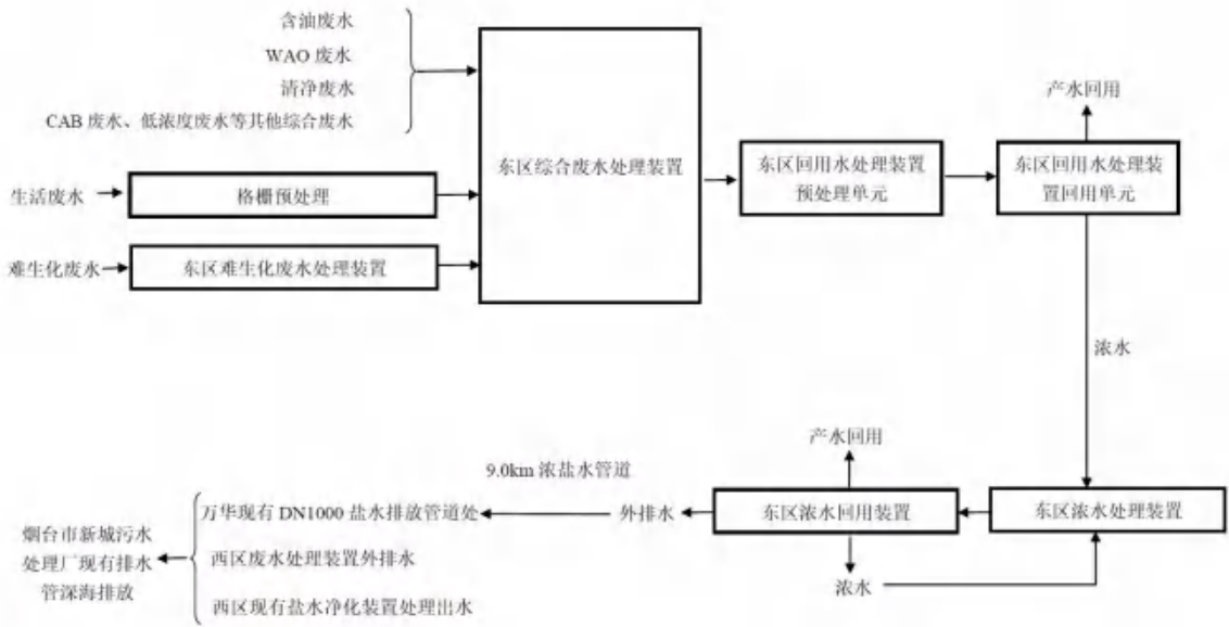
图 7.2-2 东区污水处理站总工艺流程示意图
