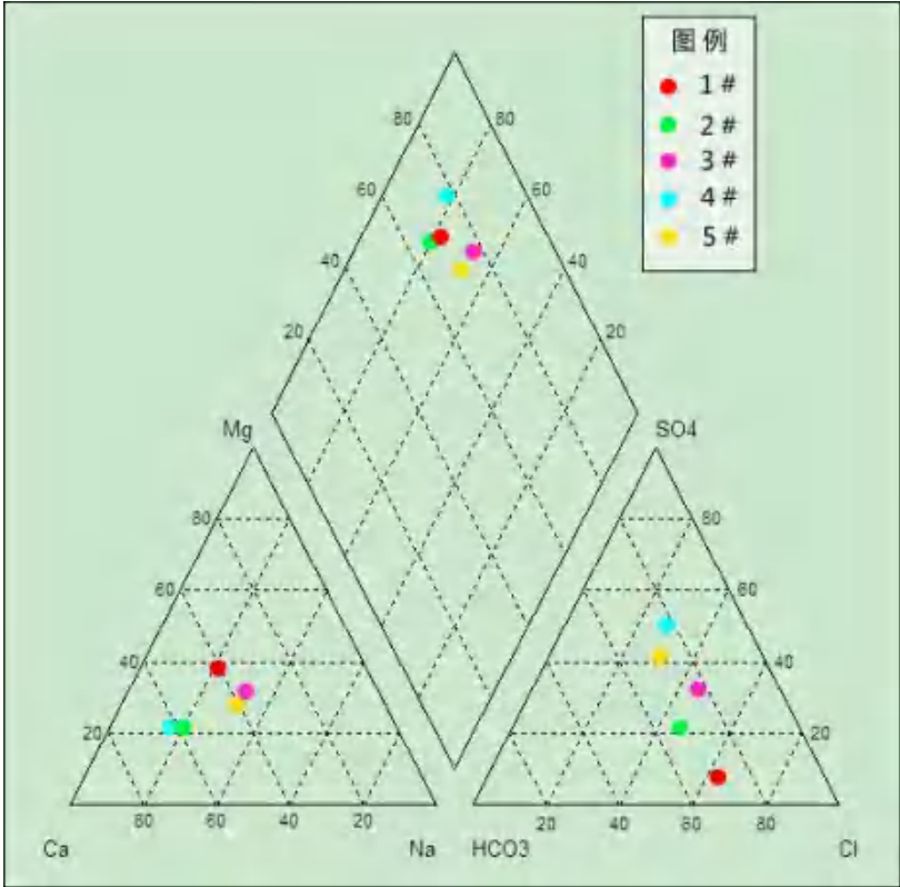
图 6.4-5 区域地下水水化学三线图
