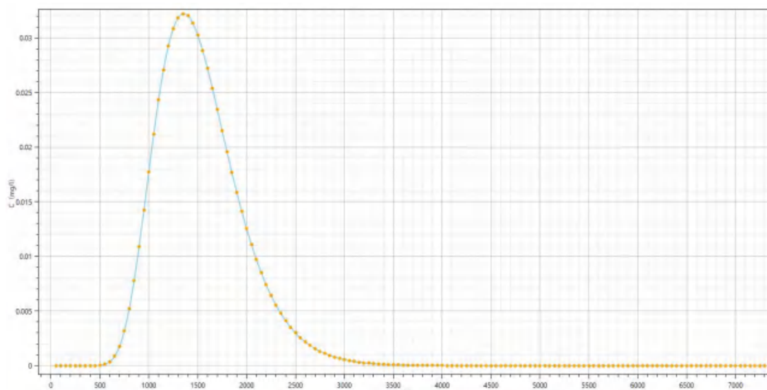
图 6.4-17 厂界浓度随时间变化关系图
