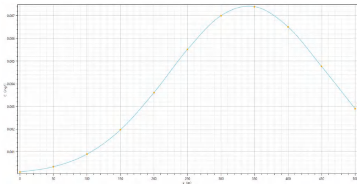
图 7.6-4 1000d 后地下水██████浓度和距离关系图
