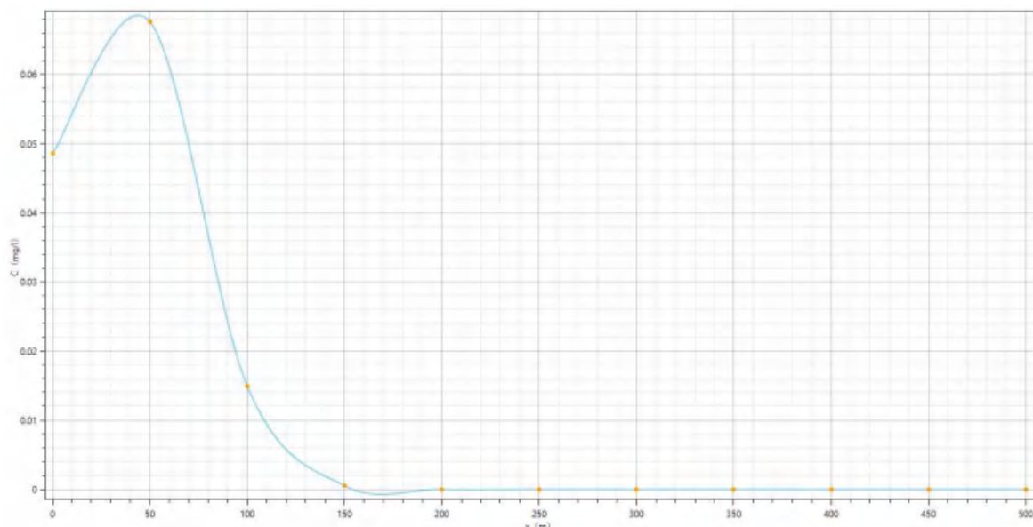
图 7.6-3 100d 后地下水██████苯浓度和距离关系图
