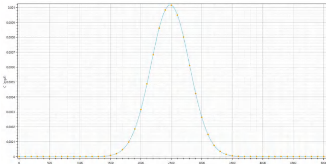
图 7.6-5 20 年后地下水■■■■浓度和距离关系图
