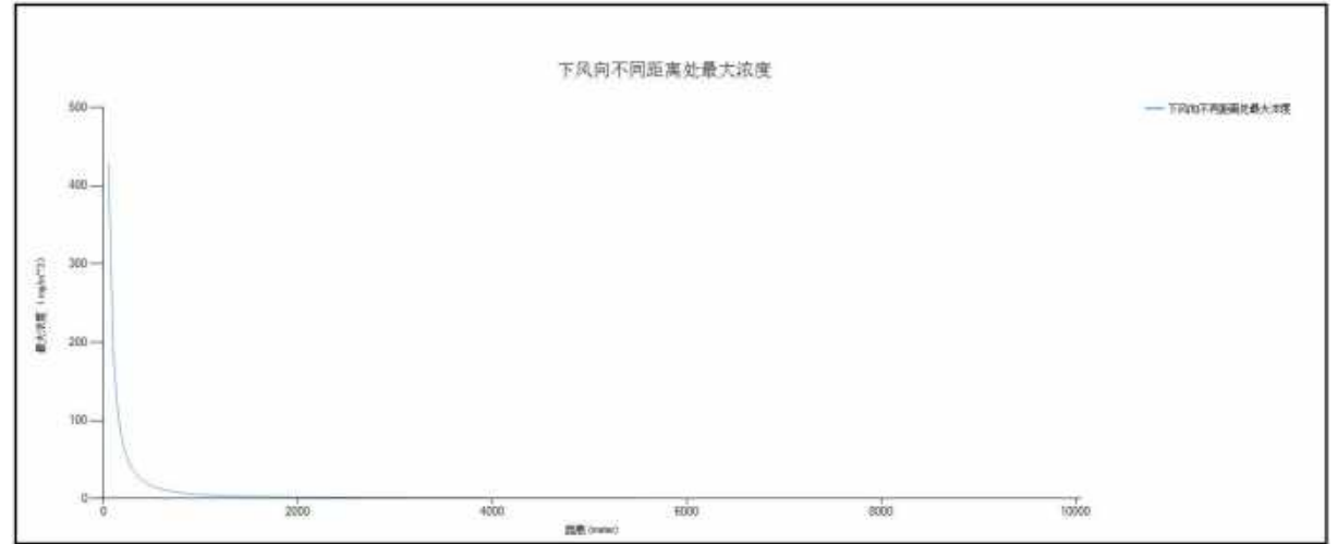
图 7.6-1 泄漏事故下风向不同距离处二甲苯的最大浓度图(最不利气象条件)
