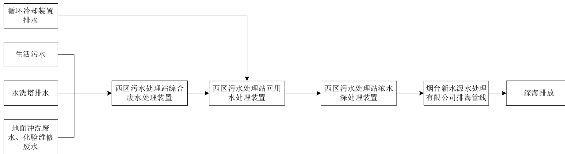
图3.12-2 项目废水处理走向图
