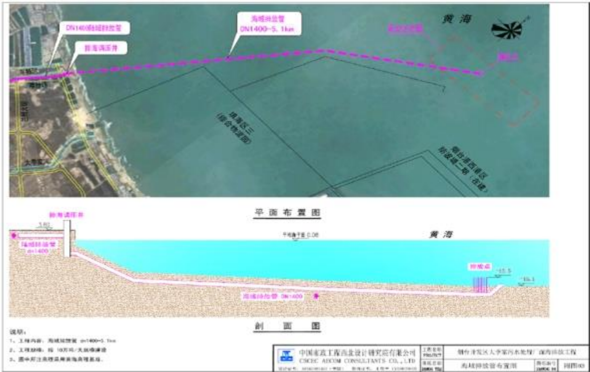
图2.2-9 新城污水处理厂排海管线工程平面布置图
