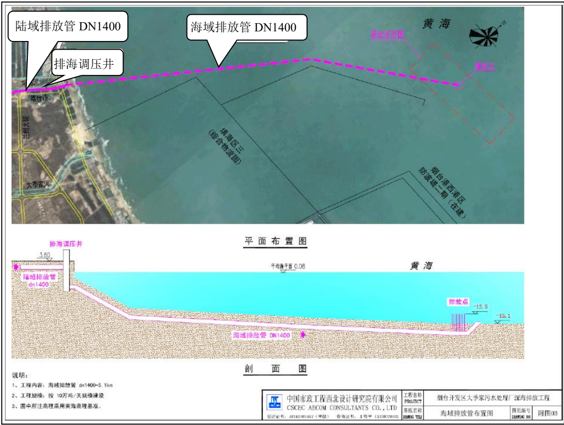
图6.3-1 依托排海管线及排海口
