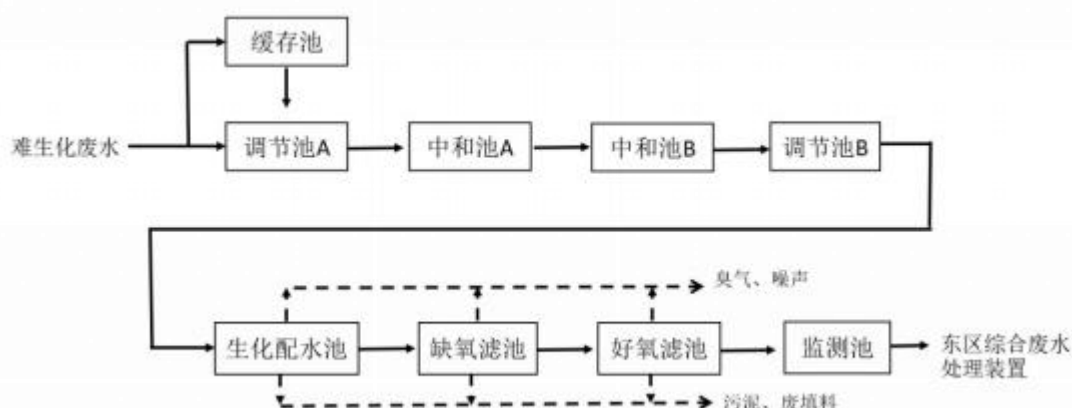
图2.2-3 东区难生化废水处理装置工艺流程及产污环节
