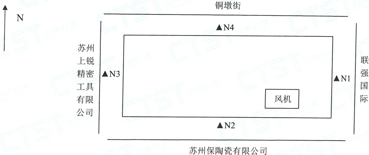
测点示意图:
