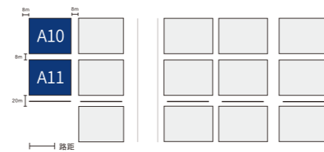
A10-A11 车间布局图 A10-A11 Workshop Layout
