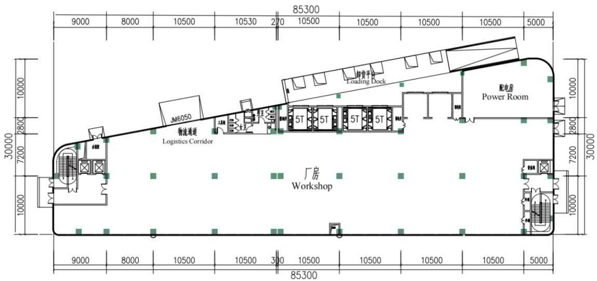
一层平面图 1 st Floor Layout
